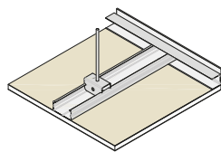
PERFIL PLADUR® T-45/T-60, HORQUILLAS, PIEZAS DE EMPALME Y CUELGUE
