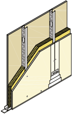
MONTANTES Y CANALES PLADUR® GAMA REFORZADA
